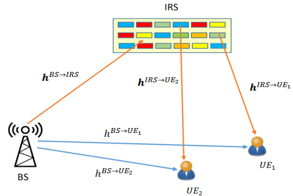
Fig. 1: IRS-NOMA system.
